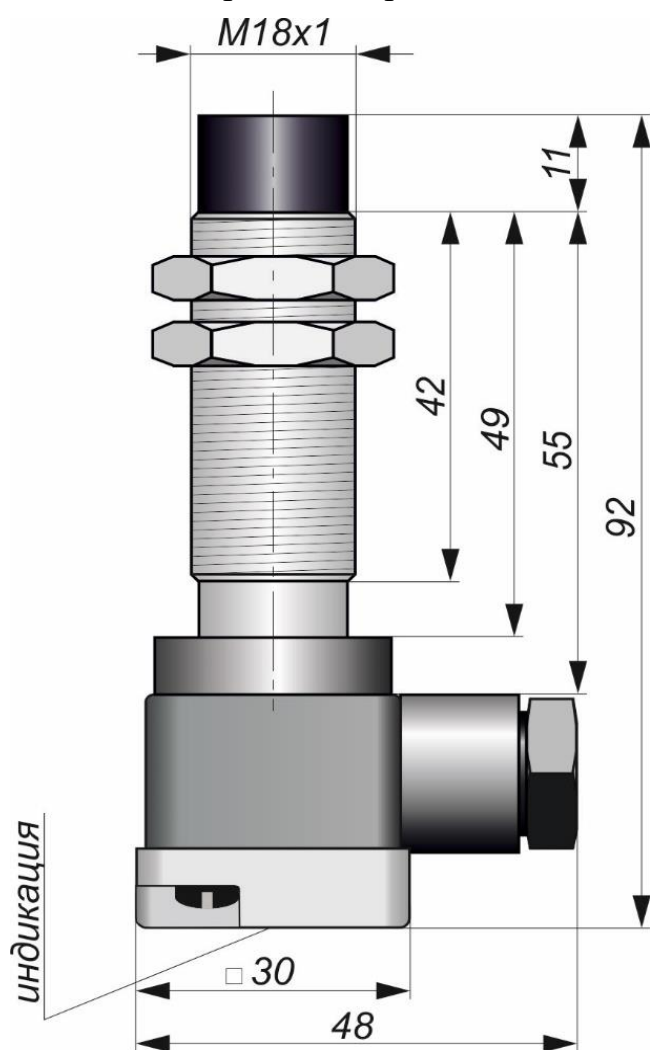
Габаритный чертеж
